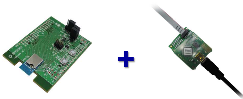
Figure 3: ホシデン製モジュール評価キット HAA0041-010030
