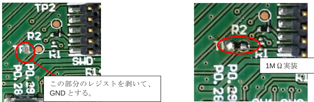
Figure 19 1MΩ 実装例
