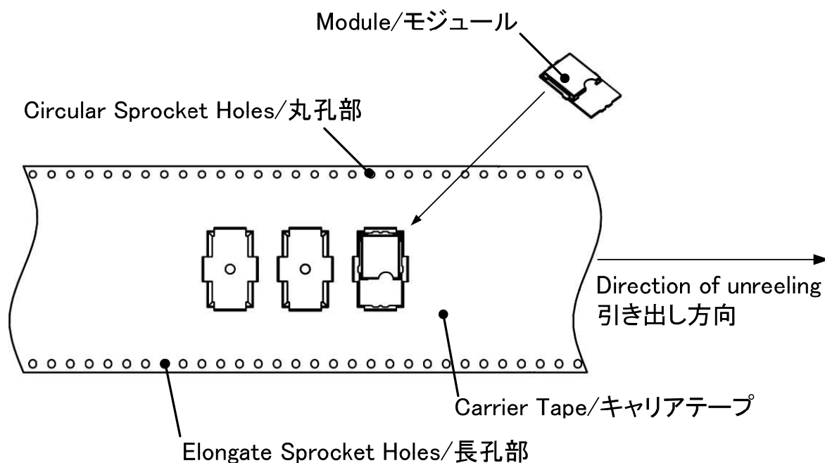
Figure 10: モジュールのテーピング条件(1)
